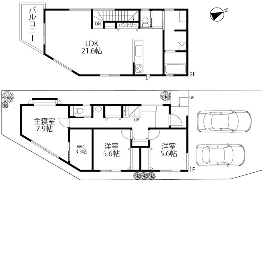
【間取り図】
